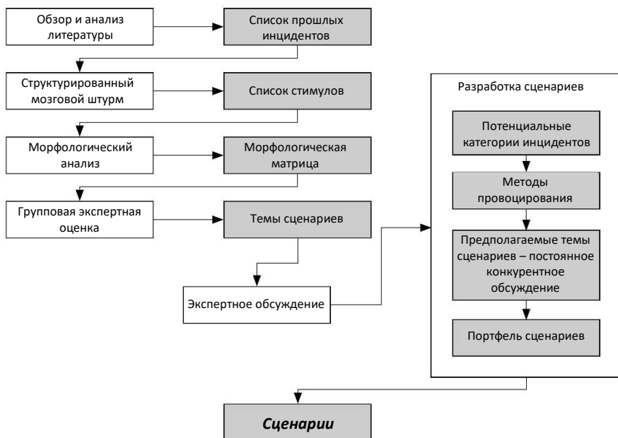
Рис. 1: Методологическая основа.
